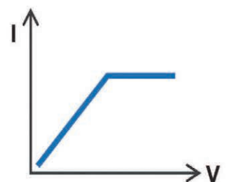
CR+CC 模式
