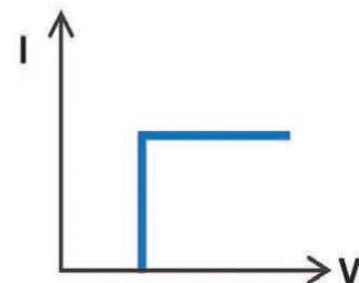
CV+CC 模式
