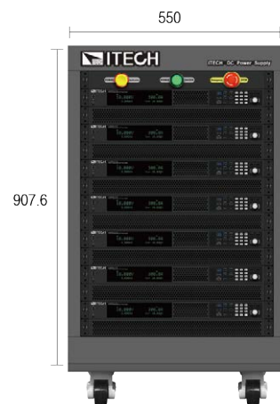
IT-E4029-15U (Dimension:mm)
