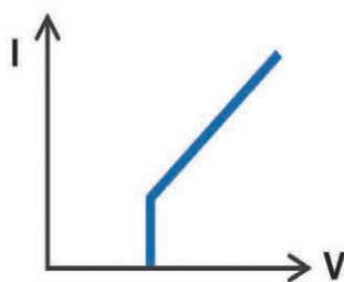
LED(CV+CR) 模式
